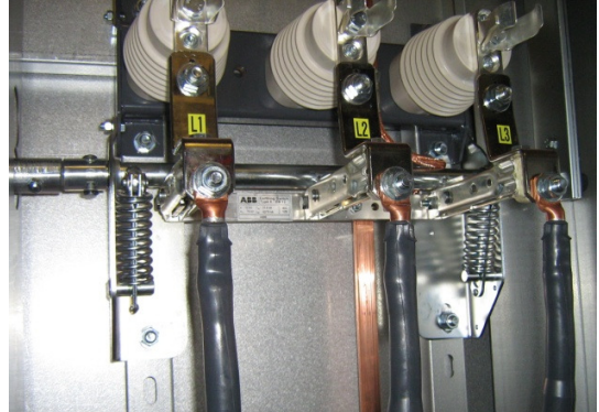
Figur 4. Jordningskopplare.
