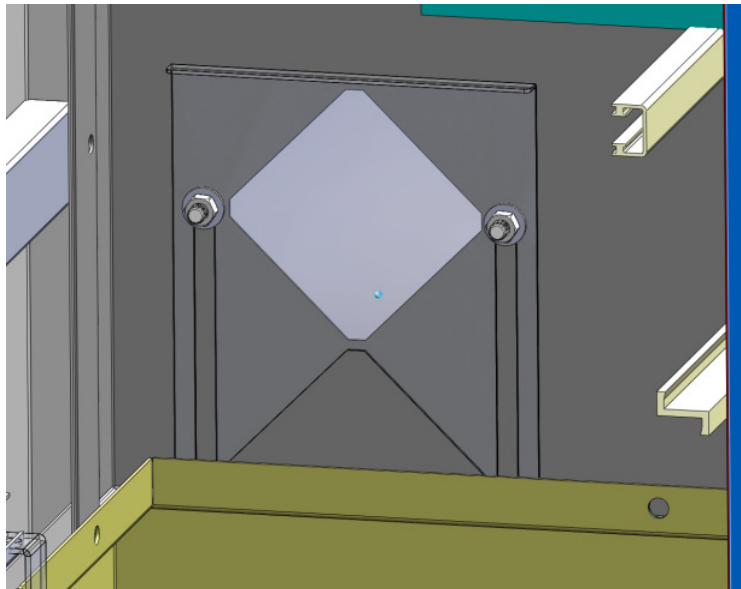
Figur 10. Reservkraftslucka.
