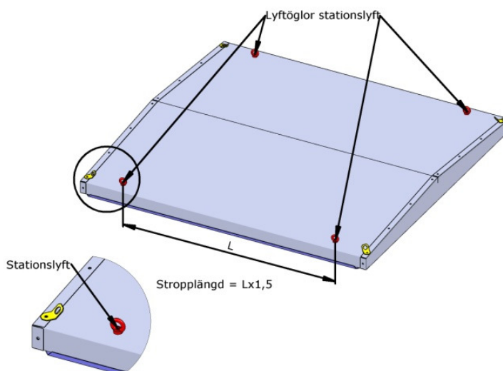
Figur 1. Stationslyft.
