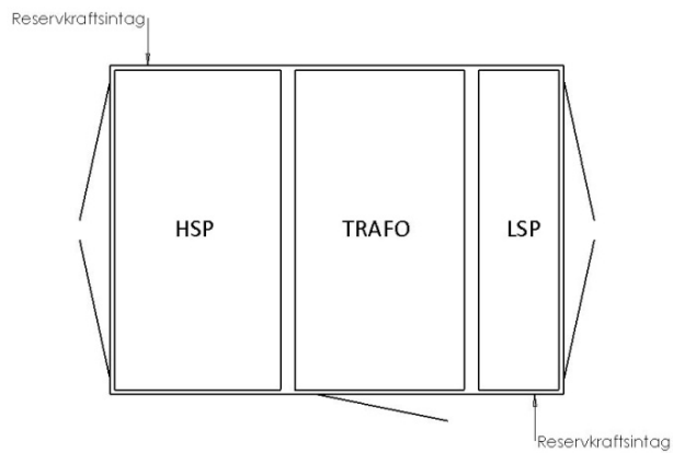
Figur 9. Reservkraftsintag Z28-RMU
