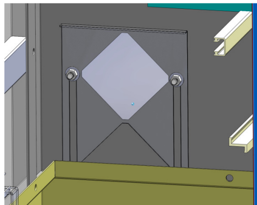
Figur 11. Reservkraftslucka.
