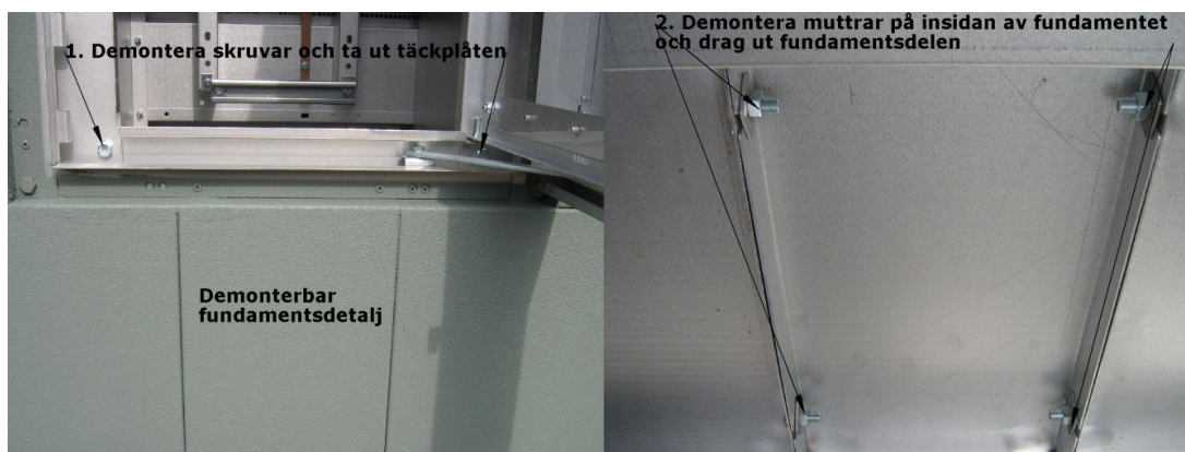
Figur 9. Instruktion kabelmontage.
