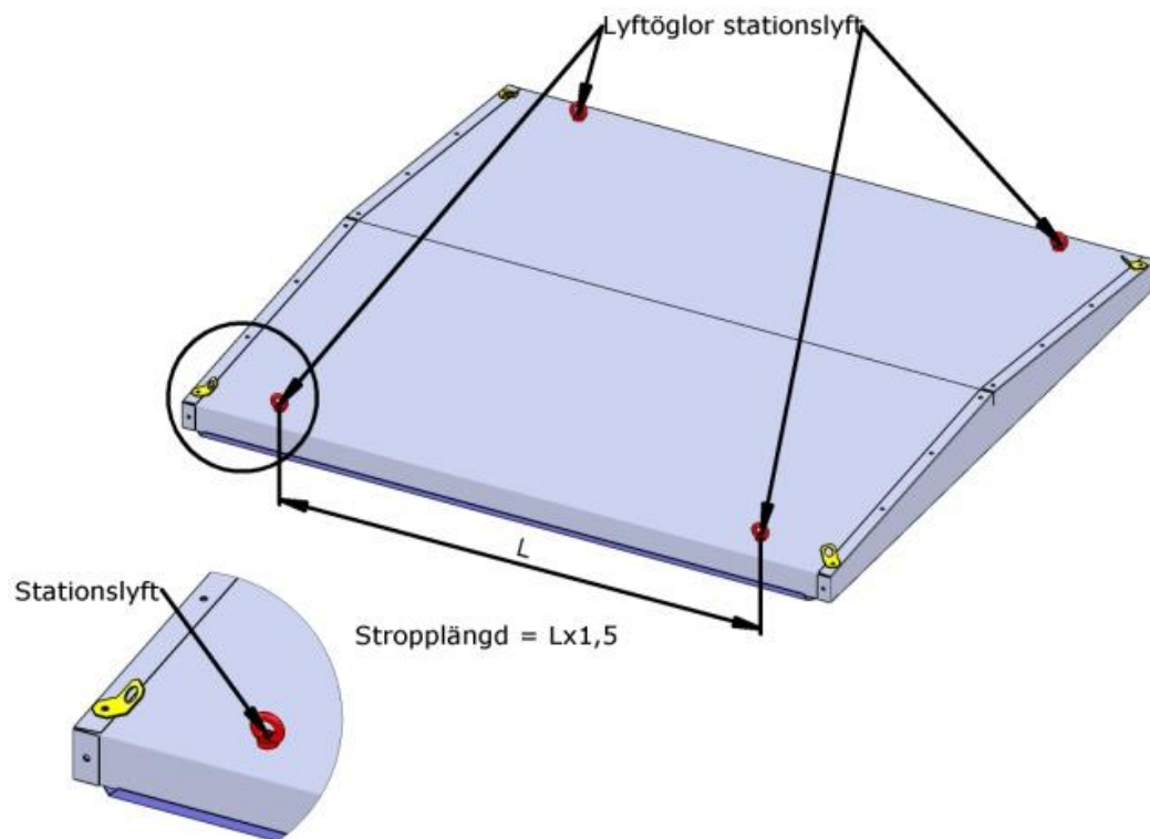
Figur 1. Stationslyft ZN22
