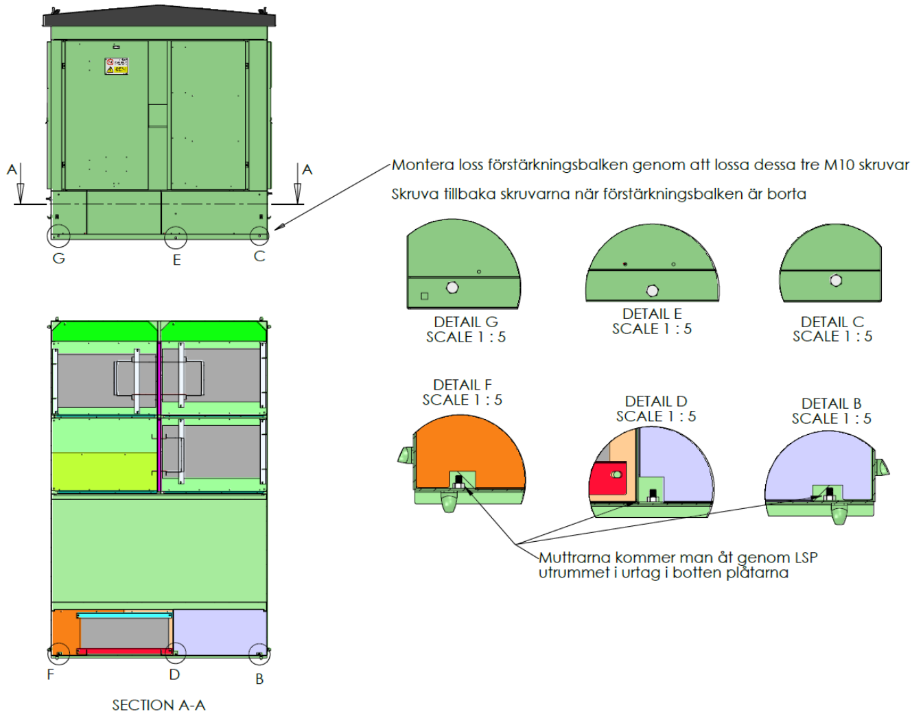
Figur 10. Kabelmontage LSP för stationer med förstärkningsbalk från ritning 53181.
