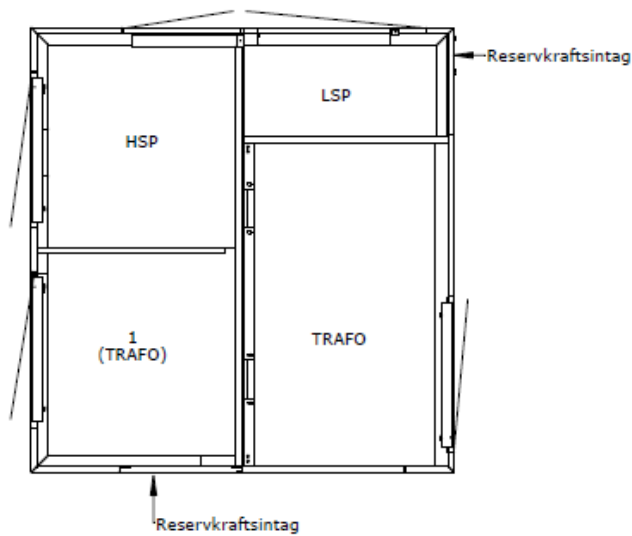
Figur 11. Reservkraftsintag ZN22.
